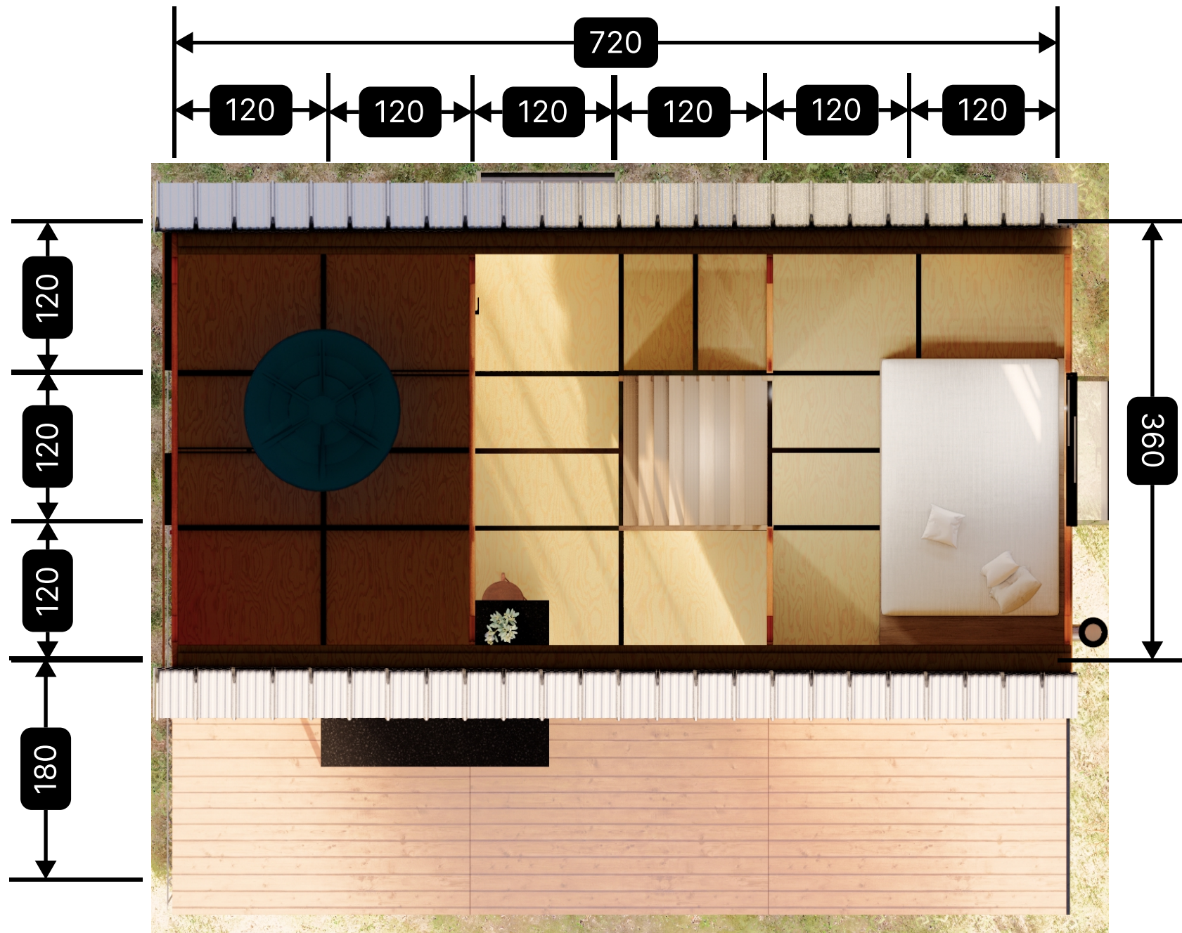
PLANTA BAIXA MEZANINO
